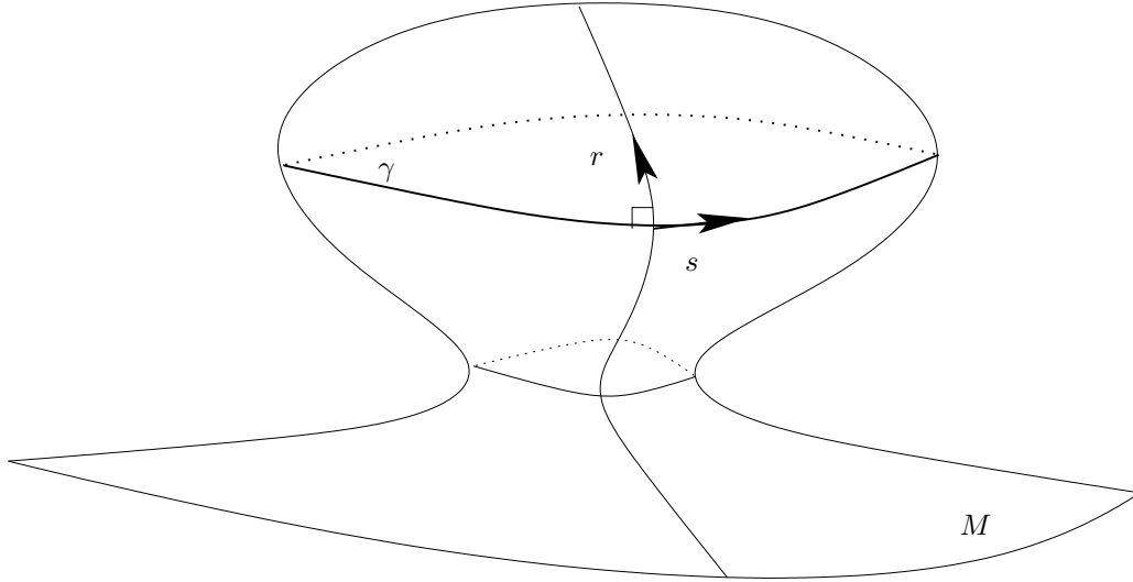
FIGURE 1 : Un exemple de surface M
