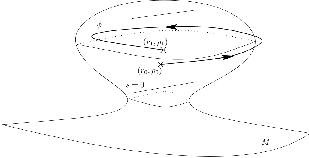
FIGURE 2 : L'application de premier retour
